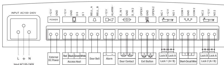
( Wiring Diagram )
